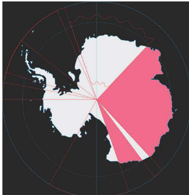
Η έκταση που έχει η Αυστραλία στην Ανταρκτική
